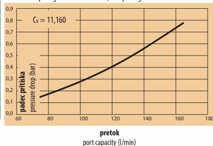
Diagram padca pritiska v vodi - DN 13, brez ventila
