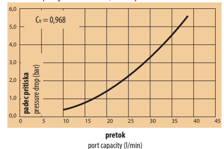
Diagram padca pritiska v vodi - DN 9, 2-stranski
