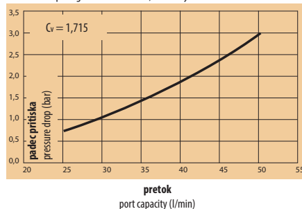
Diagram padca pritiska v vodi - DN 9, 1-stranski
