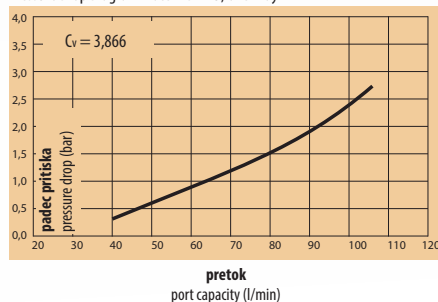
Diagram padca pritiska v vodi - DN 13, 1-stranski
