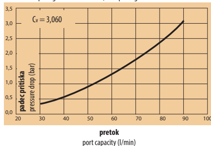
Diagram padca pritiska v vodi - DN 9, brez ventila
