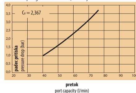
Diagram padca pritiska v vodi - DN 13, 2-stranski
